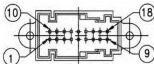
◇ 18 PIN AMP CONNECTOR : (AMP 953264-1,WHITE)
