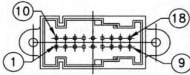
◇ 18 PIN AMP CONNECTOR : (AMP 953264-2, BLACK)
